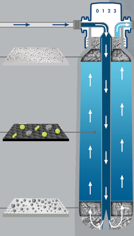
PRZEKRÓJ WKŁADU FILTRACYJNEGO BWT BESTTASTE
