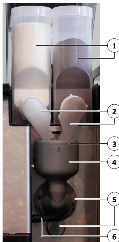
Obr. 47: Mixovací jednotka
