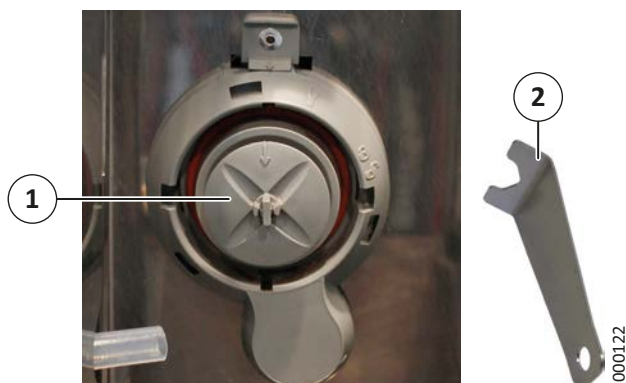
Obr. 48: Stažení kola mixéru
