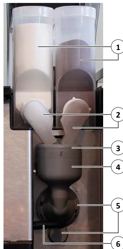
Obr. 50: Mixovací jednotka
