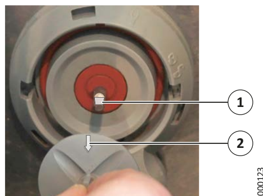
Obr. 49: Nasazení kola mixéru
